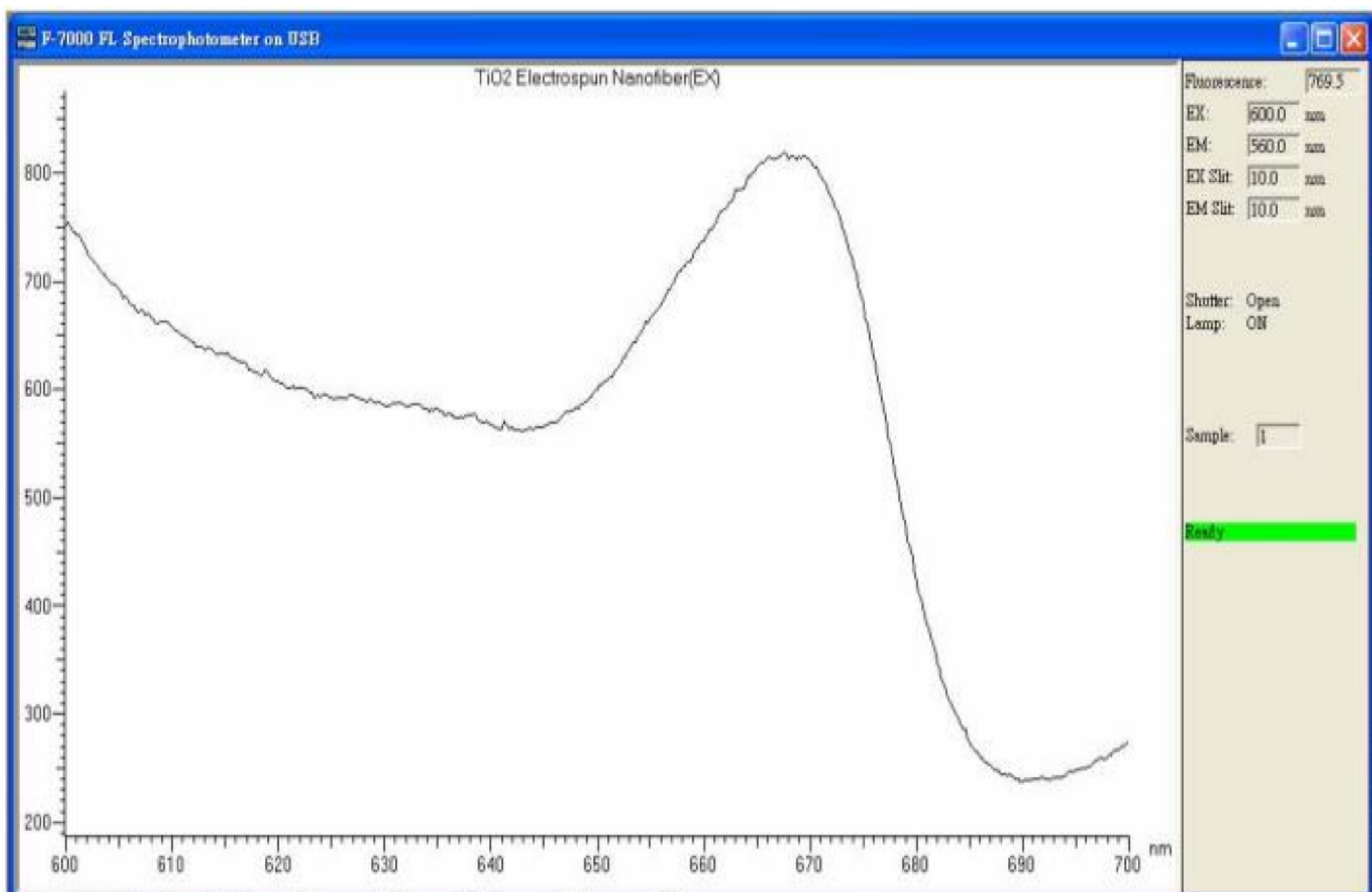
激發光譜圖
